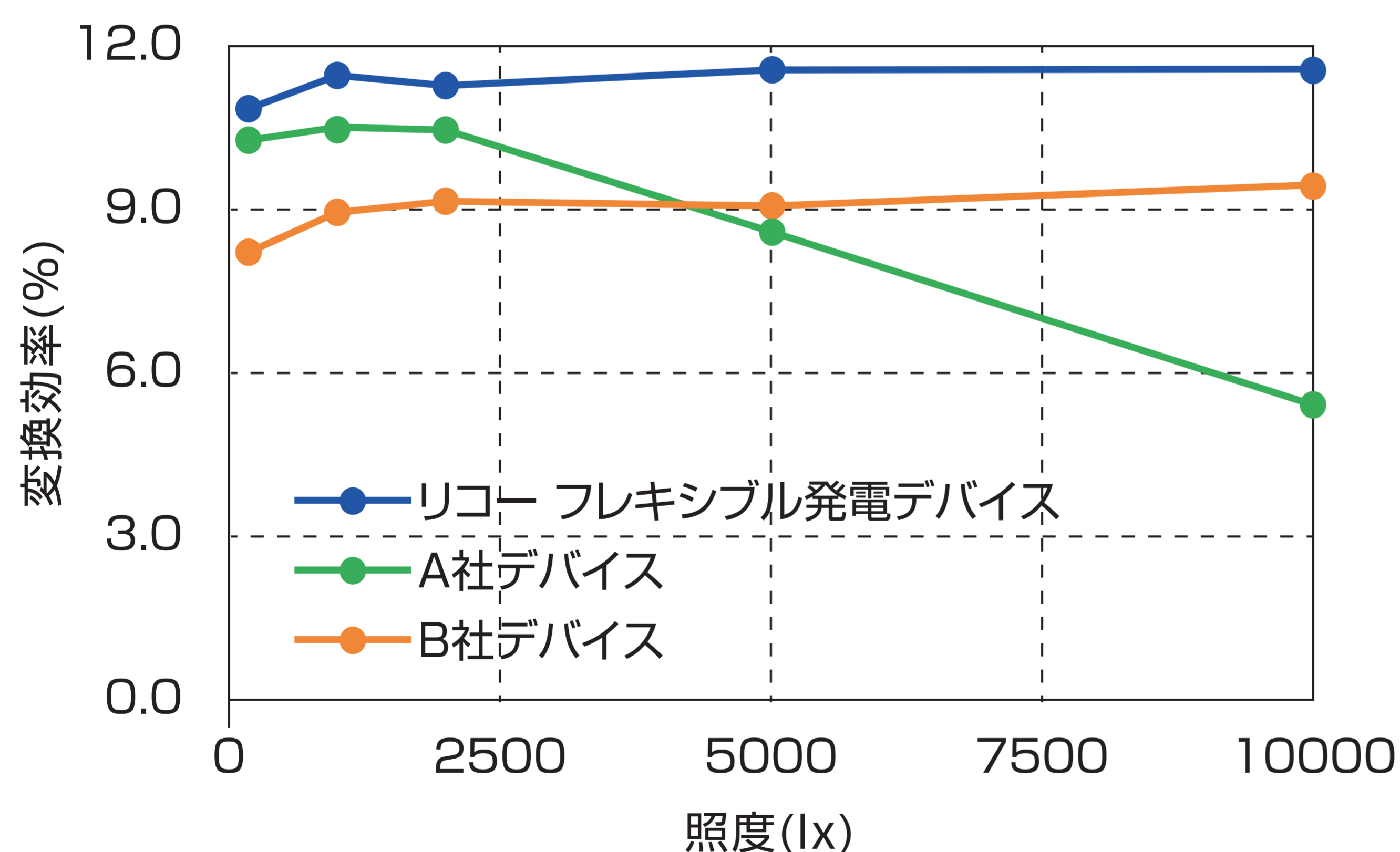
照度依存性
