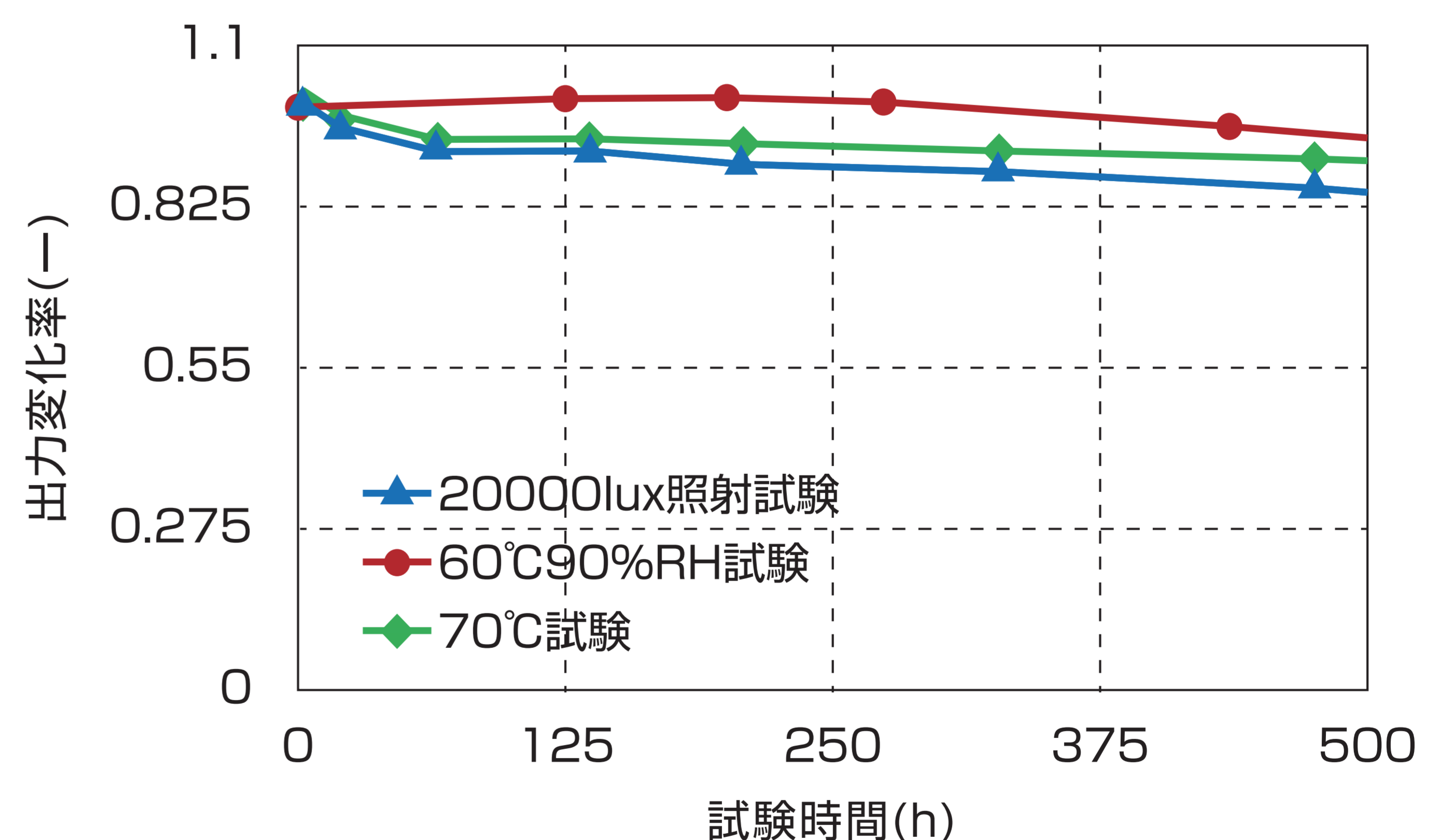
耐久性
