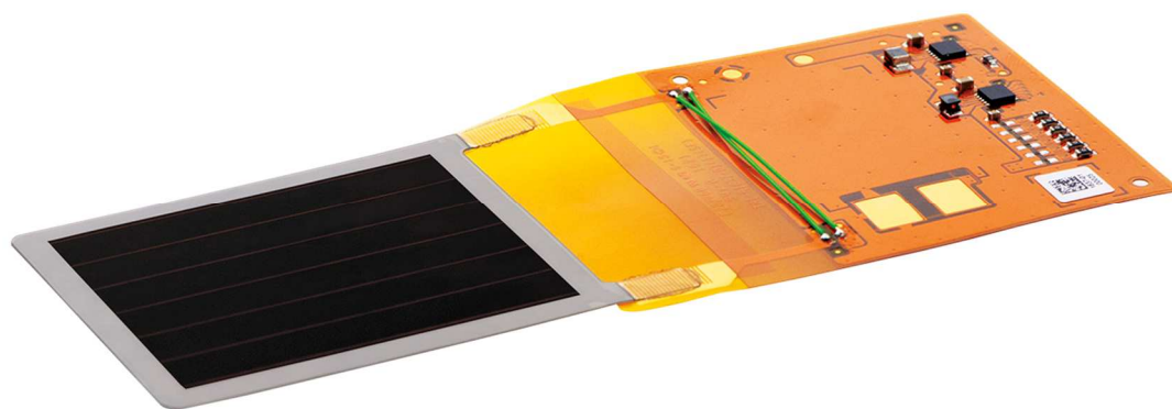
フレキシブル電源基板との接続例
